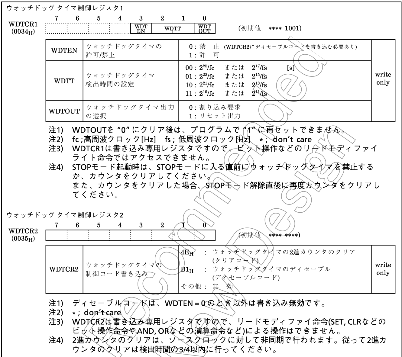
図1-28. ウォッチドッグ タイマ制御レジスタ
