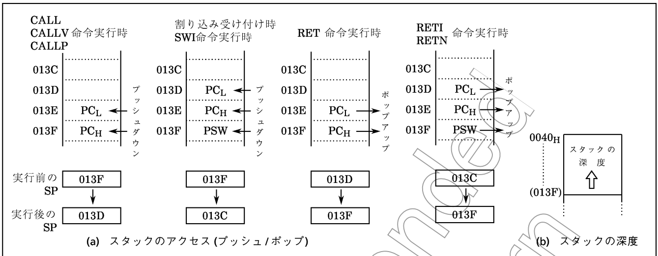
図1-8. スタック
