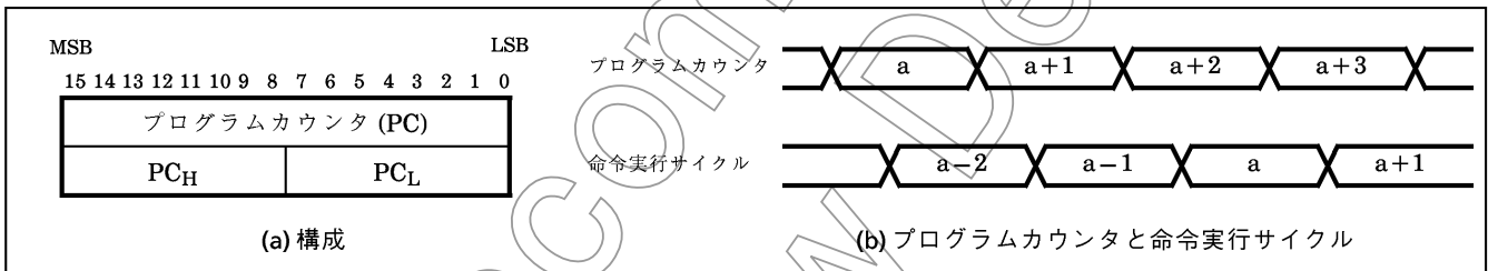
図1-3. プログラムカウンタ
