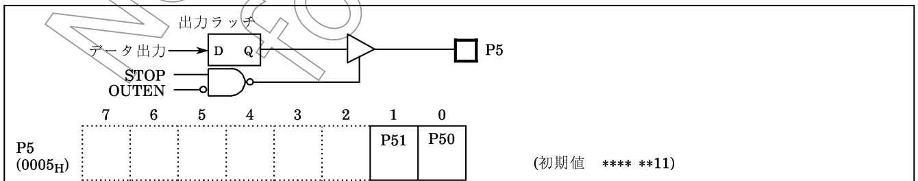
図2-6. P5ポート
