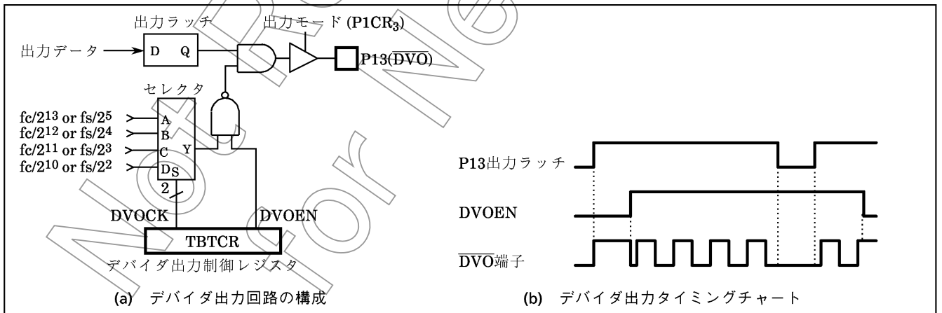
図2-12. デバイダ出力
